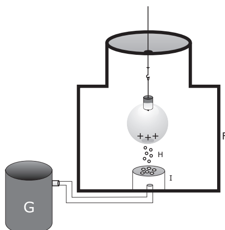
Figura 122: Representação esquemática da descrição apresentada por Gray. Letra F = recipiente que pode ser evacuado, G = Bomba de ar (ou bomba de vácuo), H = pequenas lâminas de latão sendo atraídas pela esfera de vidro eletrizada quando há uma pequena distância entre a esfera e as lâminas, I = suporte coberto com papel sobre o qual são colocadas as lâminas de latão.
