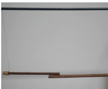
Figura 168: Em detalhe a figura apresenta duas varetas de madeira na posição horizontal presas à haste horizontal de ferro do suporte de madeira. A vareta da esquerda com uma rolha de cortiça à sua ponta está presa por linha de seda à haste e a vareta da direita está presa por linhas de poliamida (linhas de pesca).
