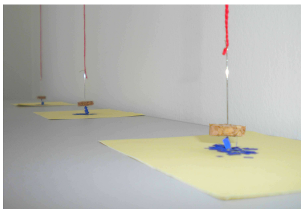
Figura 93: Os três discos de cortiça presos a linhas de algodão por meio de agulhas de costura atraindo pedacinhos de papel de seda colocados sobre um pedaço de papel sulfite após a eletrização do tubo de PVC por meio de atrito com poliamida.
