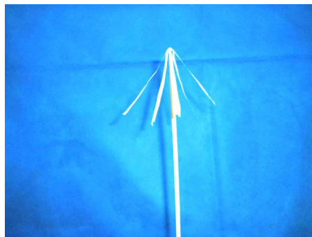
(b) Estrela (com tirinhas de 8 cm) levantada de forma radial após a aproximação do tubo de PVC eletrizado com poliamida. O tubo não está nas proximidades do instrumento.
