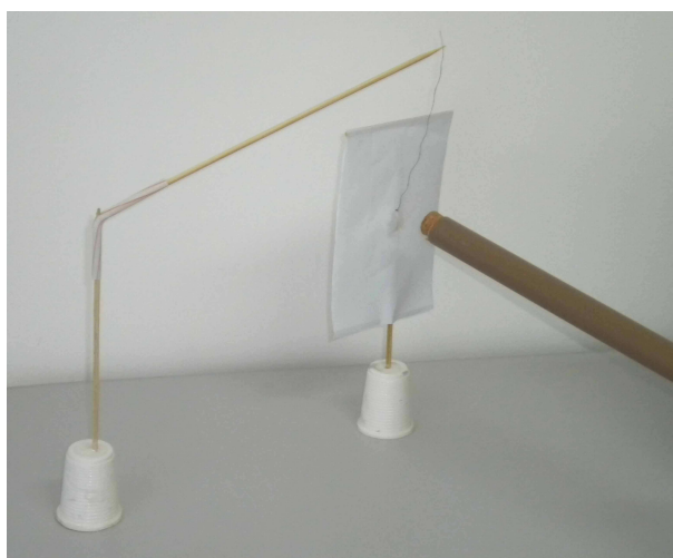
Figura 77: A penugem está presa à linha de seda ( i.e. , isolante elétrico), ao fundo temos o anteparo de papel sulfite aterrado e à frente a cortiça fixada ao tubo de PVC atritado com poliamida.
