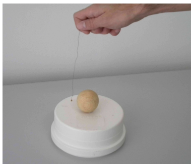
Figura 211: No alto da figura uma mão segura a linha de seda, em cuja extremidade inferior está presa uma bolinha de cortiça. A cortiça gira, no plano equatorial, ao redor de uma esfera eletrizada de madeira colocada sobre uma base de PVC atritada.
