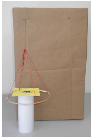
Figura 102: Aro de madeira na posição horizontal preso por quatro linhas de algodão amarradas a uma linha de seda. Esta está fixada a um palito de madeira fincado em uma caixa de papelão. A figura também ilustra os pedacinhos de papel de seda utilizados como detectores de eletrização, os quais estão posicionados sob o aro de madeira e sobre uma folha de papel sulfite. Como suporte para os papezinhos de papel de seda foi utilizado um cilindro feito com uma folha de papel sulfite.
