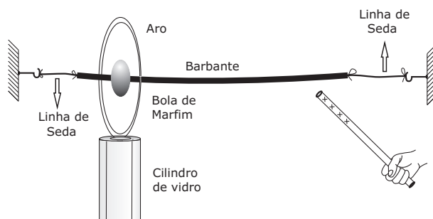
Figura 162: Barbante na horizontal, aro maior sobre o cilindro oco de vidro, bola de marfim no centro do aro, e o tubo eletrizado próximo ao barbante.
