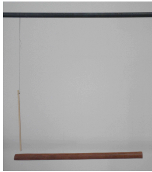
Figura 167: Em detalhe a figura apresenta a vareta de madeira horizontal presa por linhas de poliamida (linhas de pesca) na haste horizontal de ferro do suporte de madeira e a vareta vertical presa por linha de seda à mesma haste.
