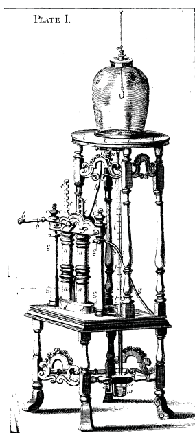
Figura 132: Gravura da bomba de ar desenvolvida por Francis Hauksbee. Extraída de (HAUKSBEE, 1709).
