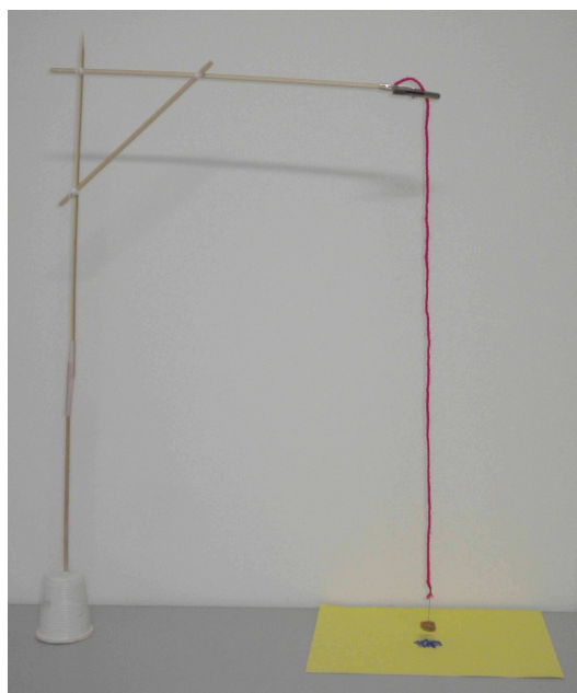
Figura 94: Aparato completo utilizado para o experimento em que há transporte de eletricidade sem que o tubo toque a linha de transmissão. Há um suporte de madeira feito com palitos de churrasco e base de gesso, uma linha de seda pendurada verticalmente ao suporte por meio de uma garra “tipo boca de jacaré” e, preso à extremidade inferior da linha, um disco de cortiça fixado por meio de uma agulha.
