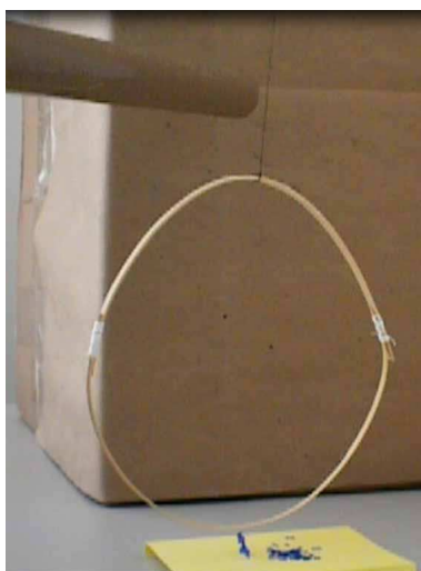
Figura 100: O aro de madeira preso a uma linha de seda atraindo pedacinhos de papel de seda colocados sobre um pedaço de papel sulfite após eletrizar o tubo de PVC por meio de atrito com poliamida e aproximá-lo da parte superior do aro.
