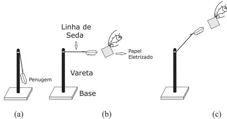
Figura 42: (a) Base, vareta e penugem pendurada por uma linha de seda. (b) Papel eletrizado (atrito) atraindo a penugem. A penugem e a linha ficam perpendiculares à vareta. (c) O papel eletrizado está além da penugem ( i.e. , mais alto do que ela) e a linha estendida como um pedaço de arame. Figura adaptada de (ASSIS, 2010, p. 83, Figura 4.21).
