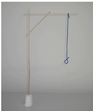
Figura 85: Aparato utilizado para sustentar o fio condutor, feito com suporte com base de gesso, palitos de madeira e linha de algodão.
