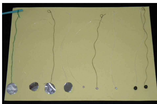
Figura 33: Alguns fios de pêndulos construídos. Da esquerda para direita - i) 4 pêndulos com disco de papel de alumínio: linha de poliamida (de “meia de seda”), linha de poliamida (linha de pesca), linha de seda, linha de algodão; ii) 3 pêndulos de bolinha de papel de alumínio: linha de poliamida (linha de pesca), linha de seda, linha de algodão; e iii) 2 pêndulos com chumbada de pesca (as menores encontradas no comércio): linha de algodão, linha de seda.
