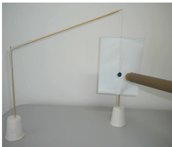
Figura 78: O disco de papel de seda (material condutor) está preso à linha de seda ( i.e. , isolante elétrico). Ao fundo temos o anteparo de papel sulfite aterrado e à frente a cortiça fixada ao tubo de PVC atritado com poliamida.
