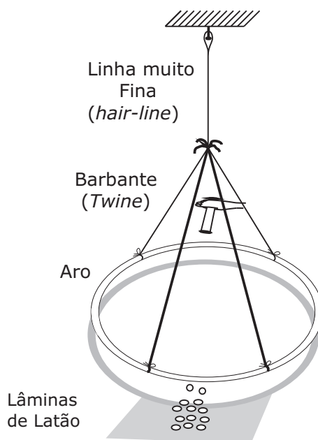
Figura 70: Ilustração do aro na posição horizontal preso a um prego no teto por meio de uma linha muito fina e de quatro barbantes. O tubo eletrizado é colocado próximo do aro, na parte oposta àquela onde estavam colocadas as lâminas metálicas abaixo de outra parte do aro. Estas lâminas são atraídas pelo aro.
