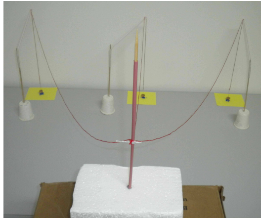
Figura 96: Aparato utilizado para o experimento em “ que a virtude elétrica pode ser transportada ao mesmo tempo por vários caminhos, por uma linha de comunicação, sem tocar a referida linha. ”. Três pedaços de linha de algodão são presos a um suporte isolado eletricamente, seguem horizontalmente até um segundo suporte isolante (suporte com base de gesso + canudo de refresco como haste horizontal) e, então, seguem verticalmente até próximo à superfície. Nesta extremidade de cada linha condutora há um disco de cortiça preso a elas por meio de uma agulha. Abaixo dos discos há pedacinhos de papel de seda colocados sobre um pedaço de papel sulfite.
