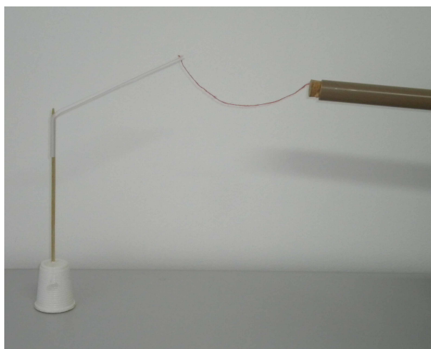
Figura 76: A figura ilustra uma linha pendular de algodão grudada em uma cortiça colocada à extremidade de um tubo de PVC após ser atritado com poliamida. A linha permanece desta forma por poucos instantes, logo em seguida é repelida pela cortiça.
