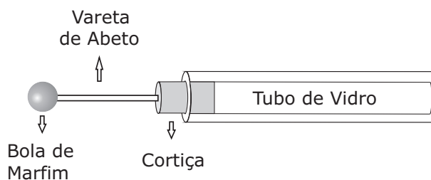
Figura 53: Tubo de vidro enrolado, vareta de abeto e bola de marfim.
