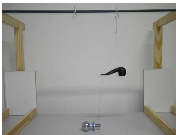
Figura 104: Aparato utilizado para suspender o cachimbo de madeira. Ao alto da figura há uma haste horizontal presa à dois suportes laterais de madeira. O cachimbo, ao centro da figura, está suspenso por uma linha isolante de seda presa à haste horizontal. Uma segunda linha de seda, presa à piteira, o prende em uma peça de ferro colocada sobre a mesa, para que o cachimbo fique na posição correta.
