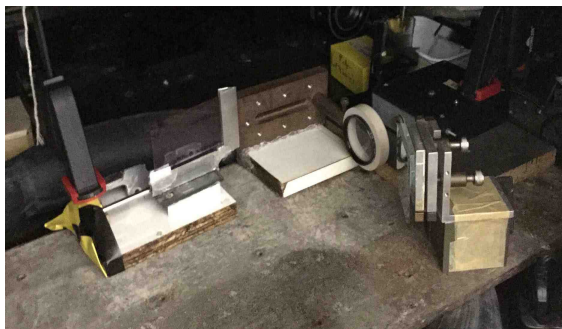
Figura 9: Parte da montagem com fonte de laser, lente convergente, suporte móvel para placa e espelho para a o feixe refratado.
