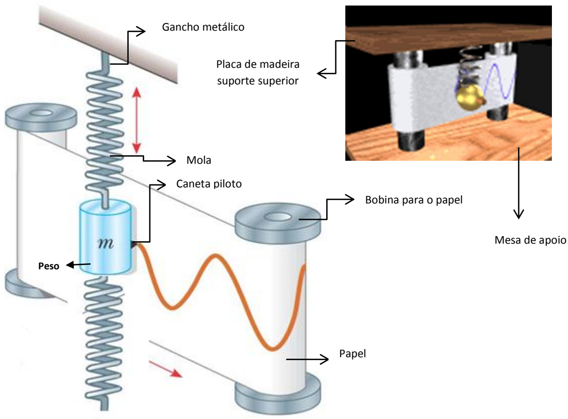
Figura 09 – Representação esquemática do dispositivo montado.
