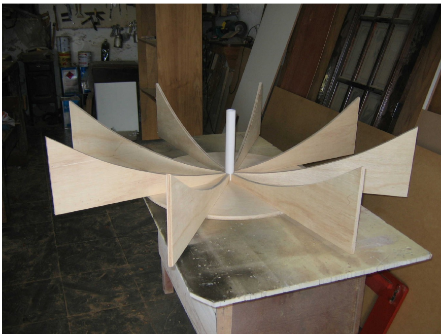
Figura 11. Espelho acústico parabólico montado (em outro ângulo).
