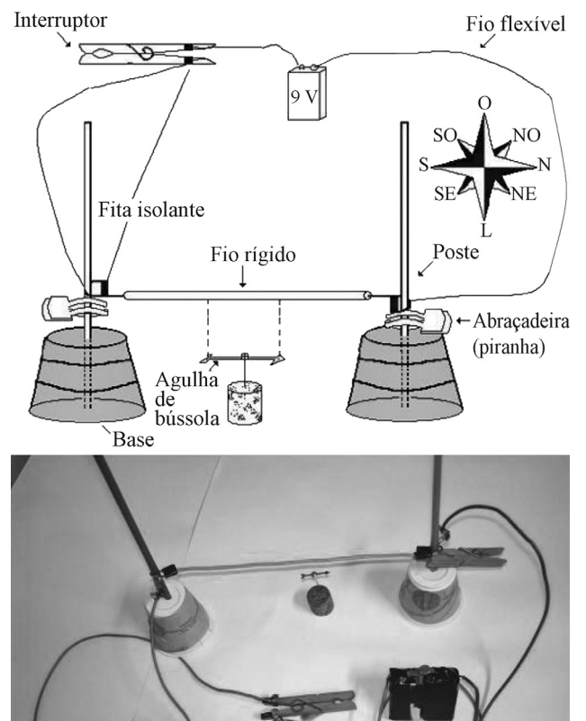
Figura 4 - O fio rígido está preso aos postes de sustentação, nivelado pelas abraçadeiras (ou pregadores) e paralelo à agulha magnética. Nesta configuração o arranjo experimental está orientado ao longo do eixo norte-sul magnético terrestre. Ao pressionarmos o pregador de roupas fazemos contato entre os condutores, fechando o circuito, e permitindo a passagem de corrente elétrica.
