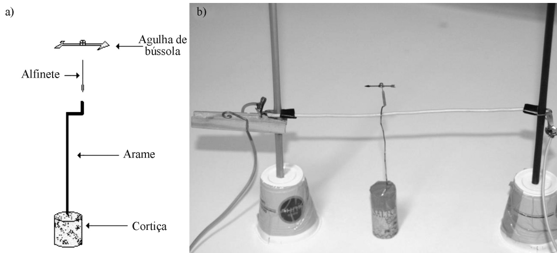
Figura 9 - A agulha magnética por cima do circuito.
