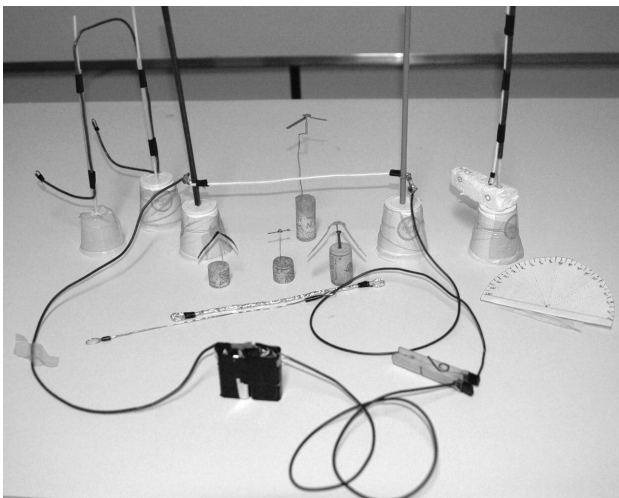
Figura 1 - Material usado para a experiência.
