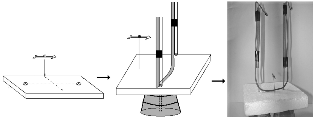
Figura 7 - Esquema para a montagem de pernas paralelas.
