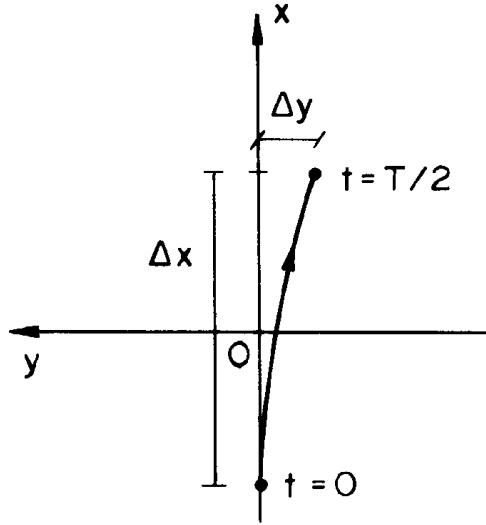
Figura 2.19: Geometria para o cálculo da precessão do plano de oscilação de um pêndulo carregado.
